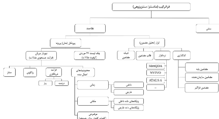
مشخص می‌نماید. در نمودار جریان‌ی پریزما چهار مرحله کلی وجود دارد که عبارتند از مرحله نحوه پیدا کردن مقالات، مرحله غربالگری، مرحله دست پیدا کردن به مقالات مرتبط و مرحله جمع‌بندی مقالات مرتبط. مرحله اول، گردآوری مقاله‌های در ارتباط با مرور، تعداد مقاله‌هایی که از راه جستجو در پایگاه داده‌ها و همین‌طور سوابق اضافی که از راه منابع دیگر به‌دست می‌آیند را شامل می‌گردد. بعد از آن مرحله غربالگری است که نشانگر تعداد مقالاتی است که پس از حذف موارد تکراری باقی می‌مانند. پس از آن متن کامل مقاله‌ها از نظر واجد شرایط بودن (شایستگی) بررسی می‌شوند و دوباره از میان این مقاله‌های کامل، مواردی با بیان دلایل (معیار خروج) حذف می‌گردند. در آخرین مرحله، بعضی از مقاله‌ها برای تهیه مقاله کیفی (مرور نظام‌مند) مورد استفاده قرار می‌گیرند.
