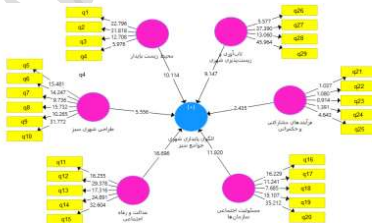
شکل ۳. مدل اندازه‌گیری اولیه در حالت معناداری ضرایب
