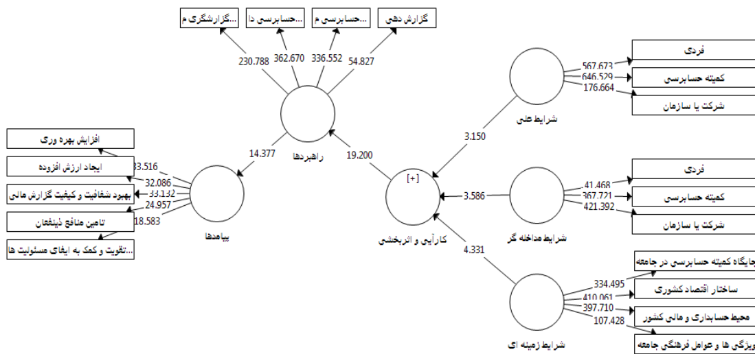
شکل ۳. ضرایب تی
