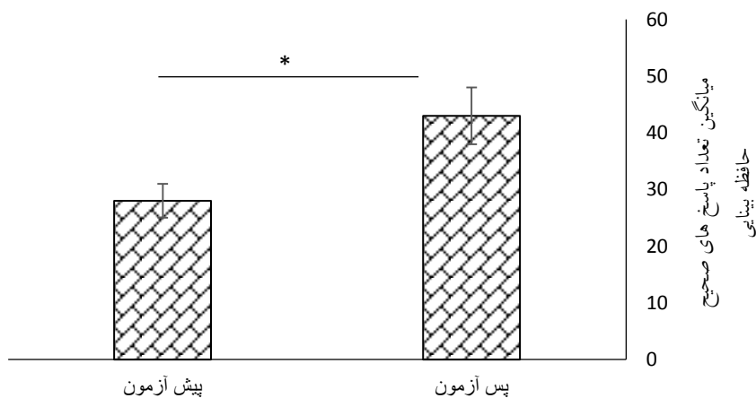
نمودار ۱. نتایج آزمون تی همبسته حافظه بینایی
