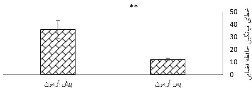
نمودار ۲. نتایج آزمون تی همبسته حافظه فضایی
